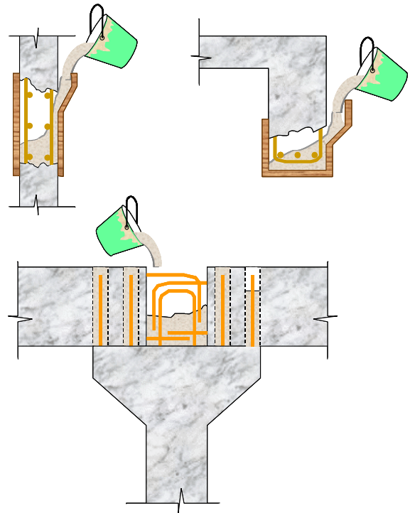
Figura 1. Grauteamento de grandes vãos confinados ou semiconfinados, utilizando Denvergrout PROTECT . No exemplo: grauteamento de bicheiras, reconstituição de seções, preenchimento de grandes juntas entre elementos estruturais, etc.
